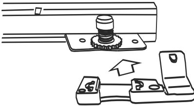
Левая направляющая
